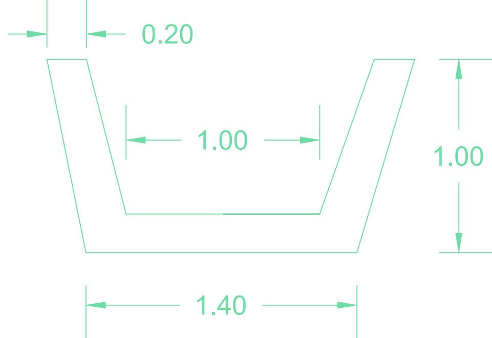
Seção do canal a céu aberto - escala 1/20
