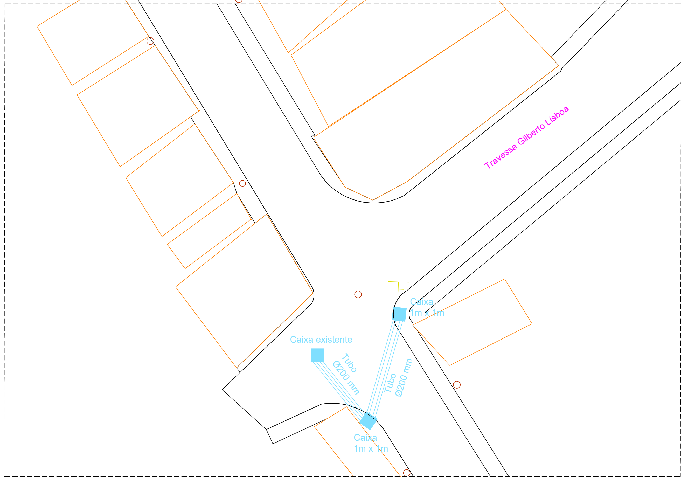
Detalhe 1 - escala 1/150
