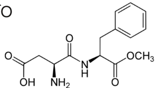
Aspartame
