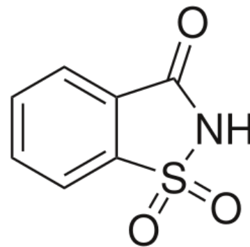
Saccharin
