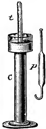
FIG. 186.—C, mercury vessel; t, eudiometer; p, pipette.
