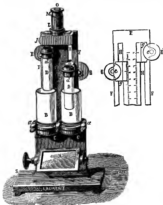
FIG. 246.—The Dubosq Colorimeter.
