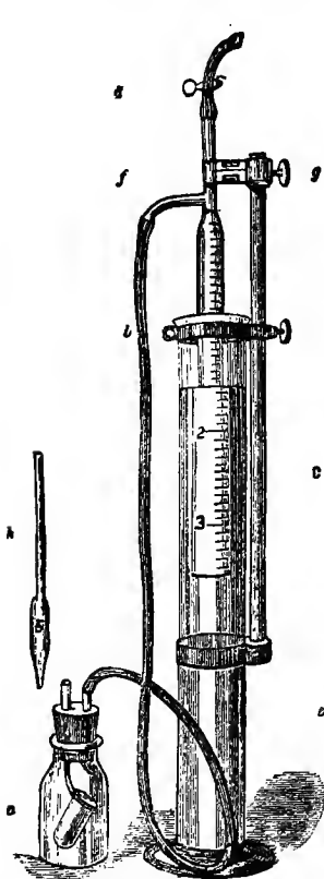
FIG. 242.—Dupré's urea apparatus.
