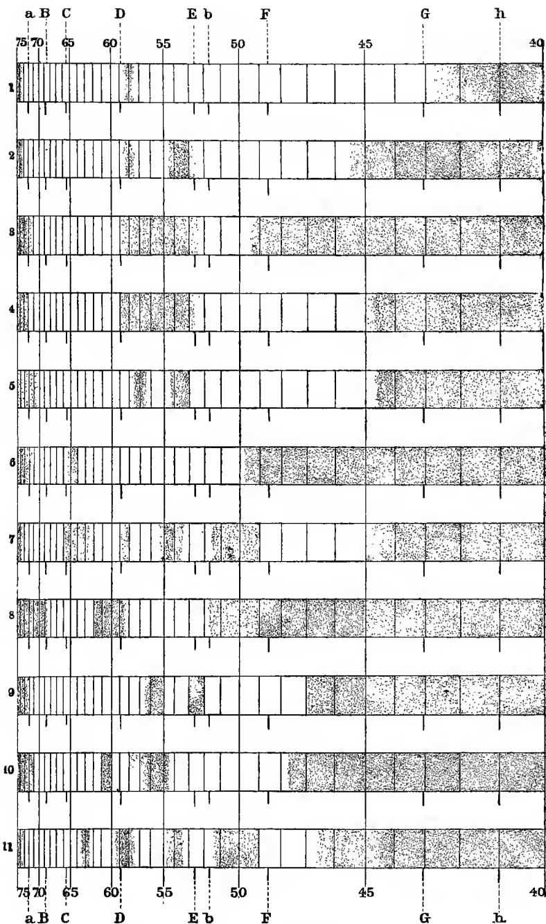
FIG. 2.1.—Absorption spectra.
