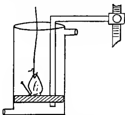
FIG. 94.—Heart chamber.
