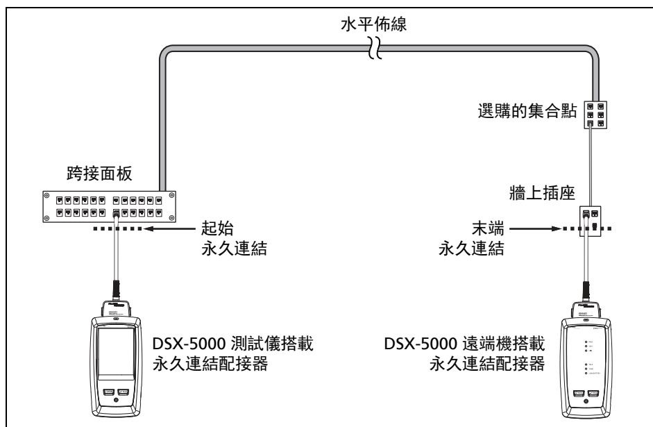
圖 3. 永久連結連接
