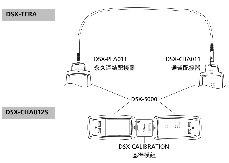
圖 2。Class F A 測試極限值基準連接
