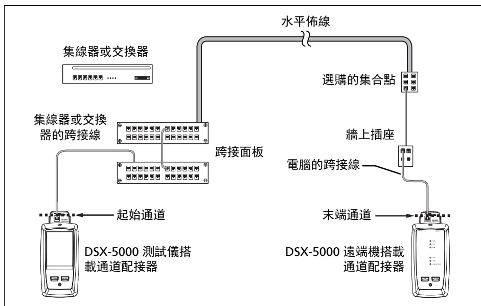
圖 4. 通道連接 (顯示 DSX-CHA012 通道配接器)
