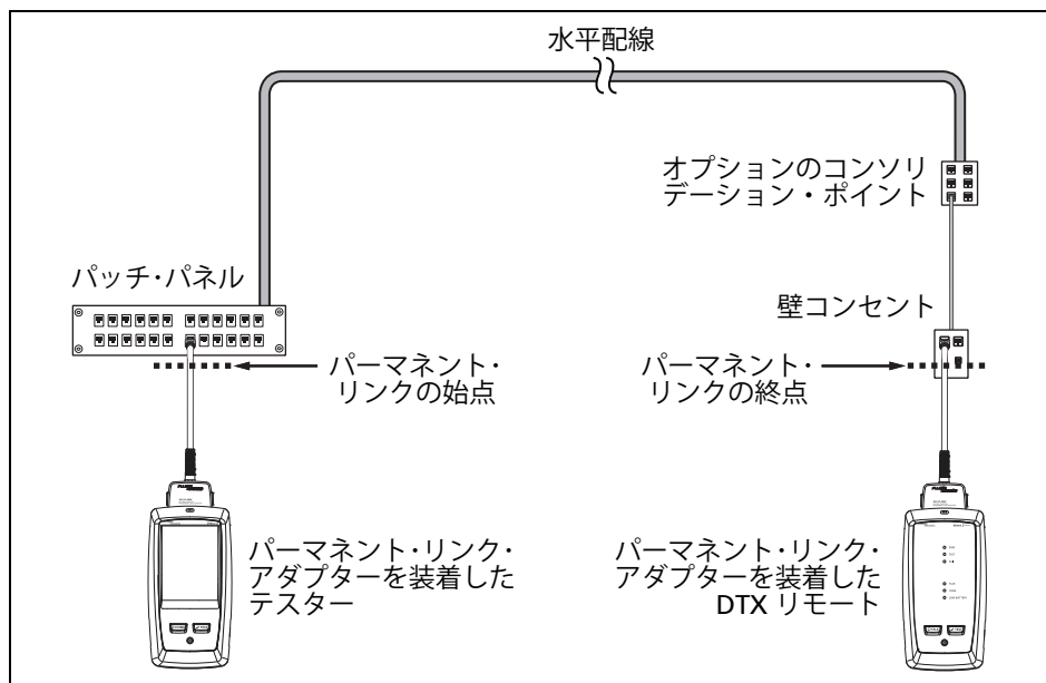
図 2. パーマネント・リンク接続
