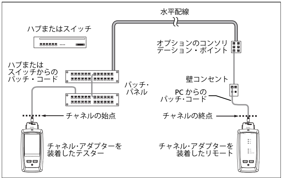
図 3. チャネル接続
