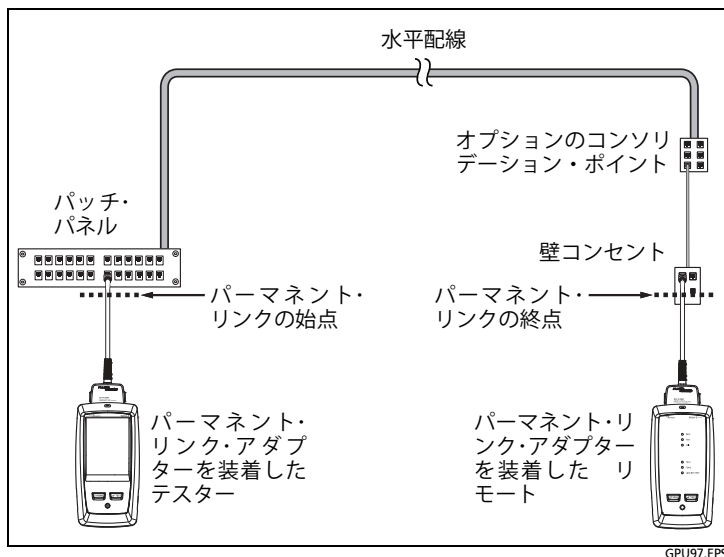
図 3. 最大で Cat 7 A のリンク用のパーマネント・リンク接続
