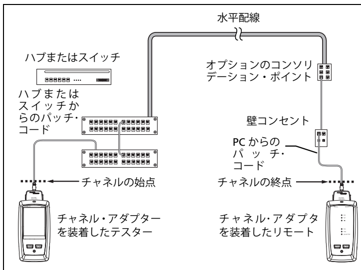
図 4. 最大で Cat 7 A のリンク用のチャンネル接続
