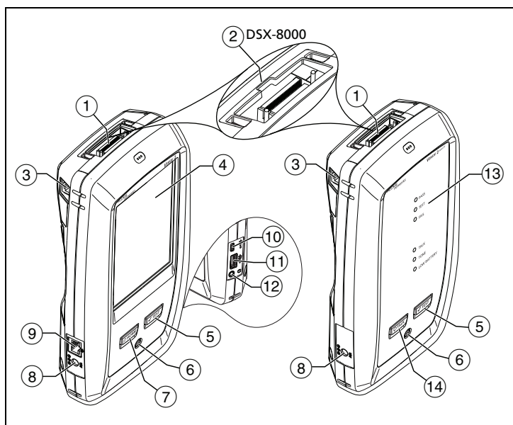
図 1. コネクター、キー、LED (Versiv 2 を表示)
