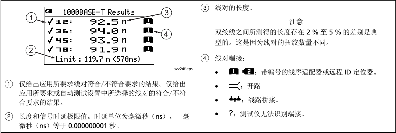
图 12. 长度结果屏幕
