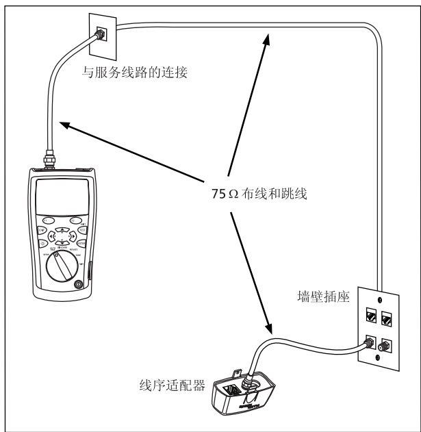
图 13. 同轴电缆布线的自动测试连接
