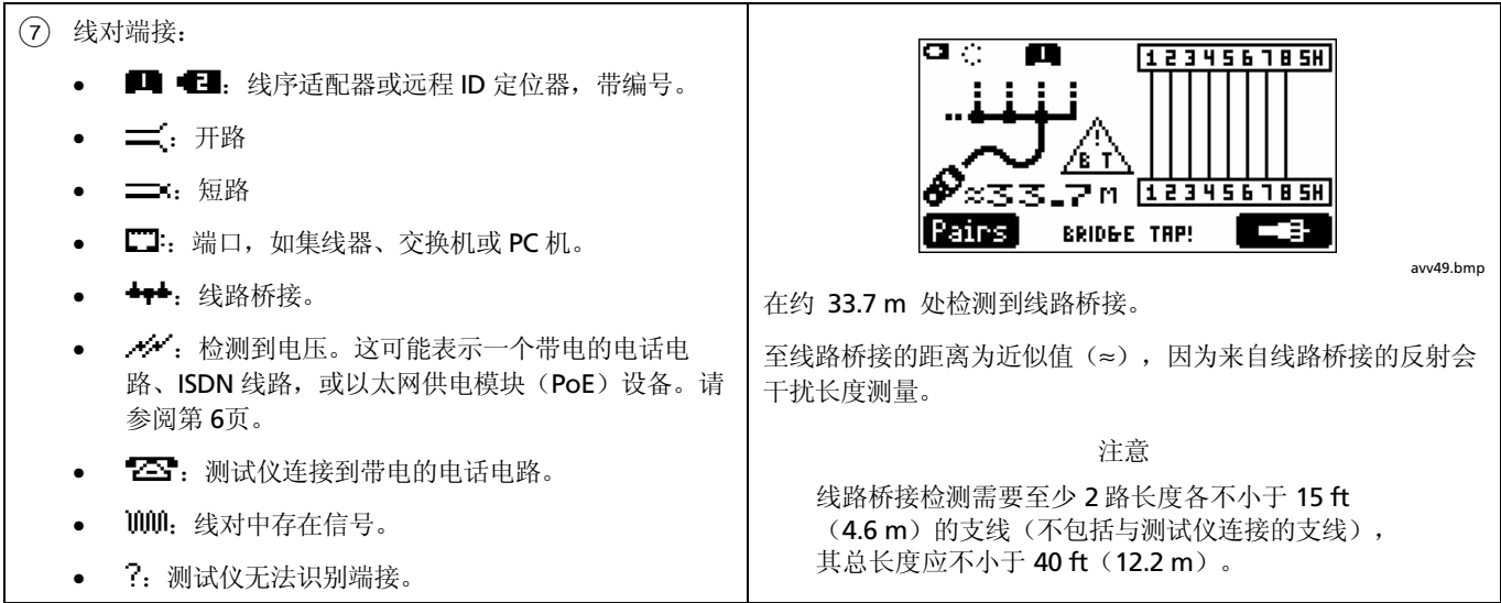
图 15. 双绞线布线的检测模式结果 (续)
