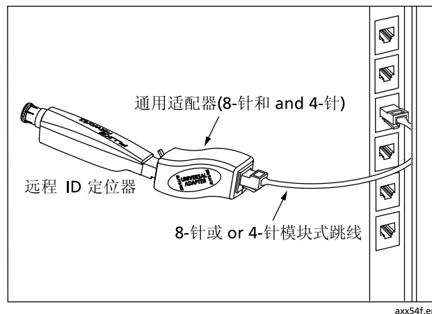
图 3. 在狭窄区域中使用通用适配器
