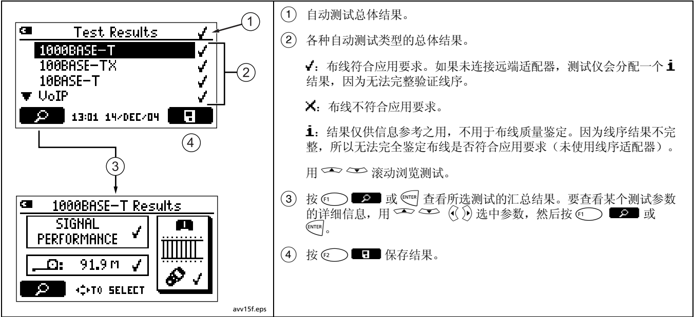
图 9. 自动测试汇总屏幕
