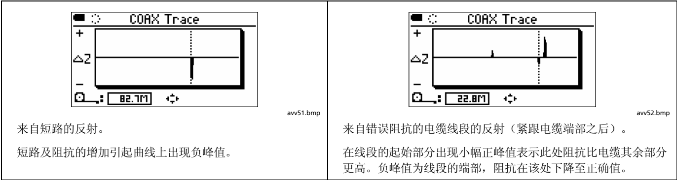
图 17. 同轴电缆布线的 TDR 绘图（续）
