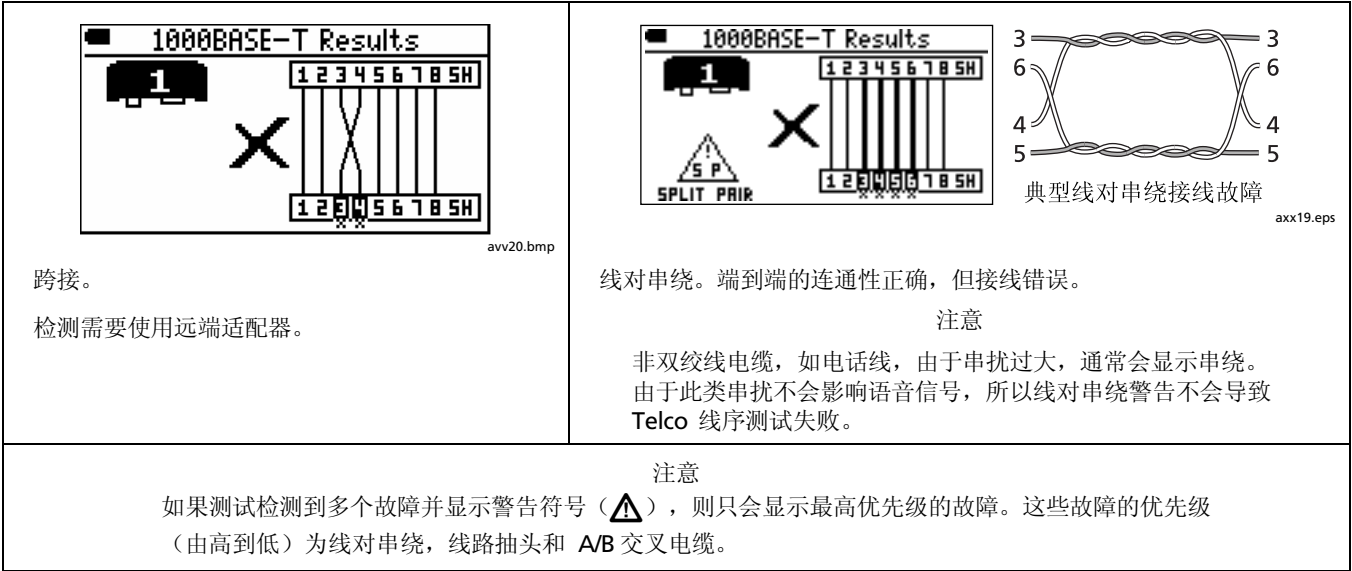
图 10. 典型线序显示（续）
