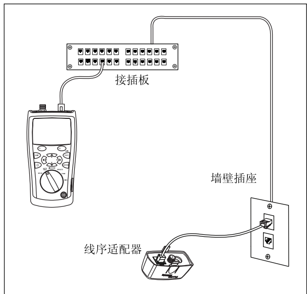
图 6. 双绞线网络布线的自动测试连接
