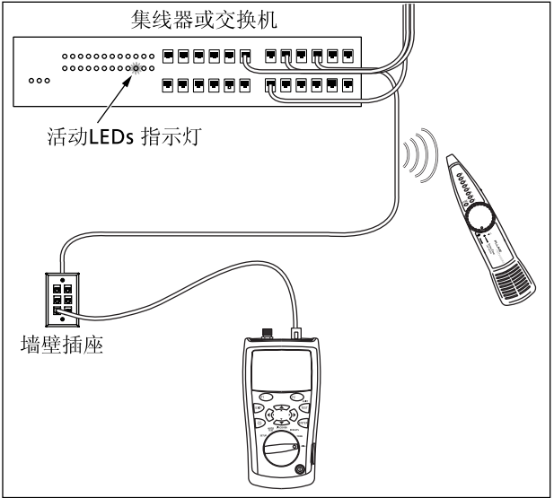
图 22. 使端口指示灯闪烁
