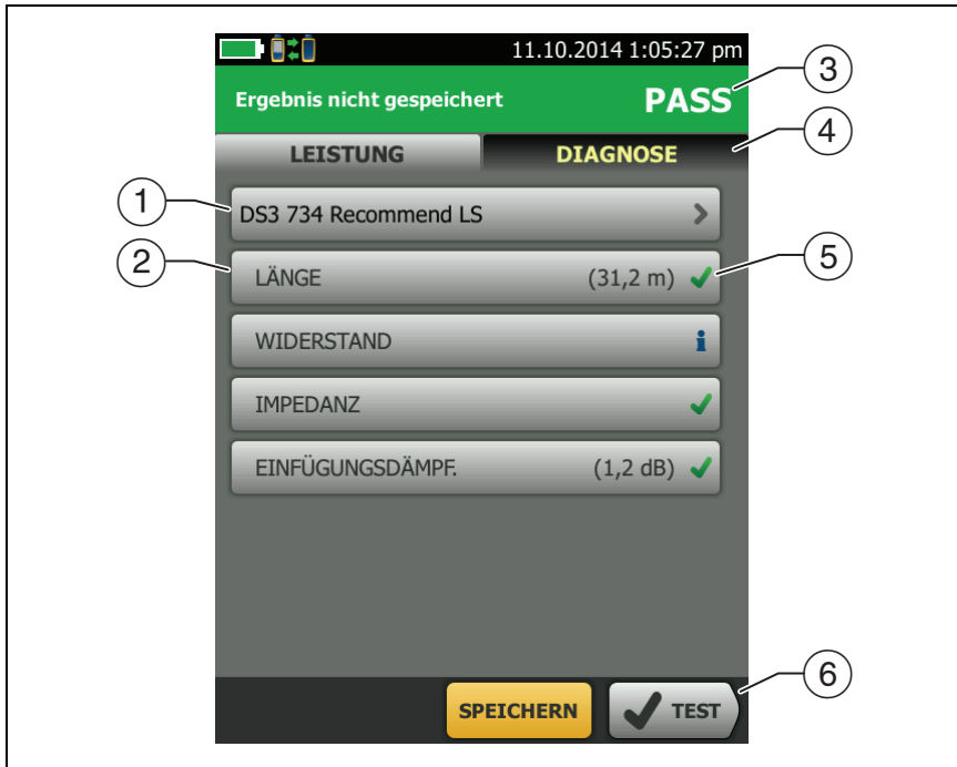
Abbildung 25. Autotest-Ergebnisse für Koaxialverkabelung
