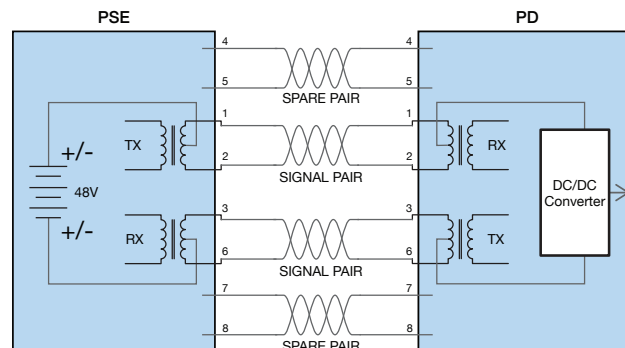
Méthode A. compatible avec 10/100/1000BASE-T et transmet simultanément la puissance avec les données en s'appuyant sur un branchement centré du transformateur.
