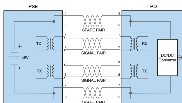
Méthode B. qui profite des paires en trop dans les câbles Ethernet à paires torsadées, est une approche facile mais qui n'est compatible qu'avec les applications 10/100Base-T.
