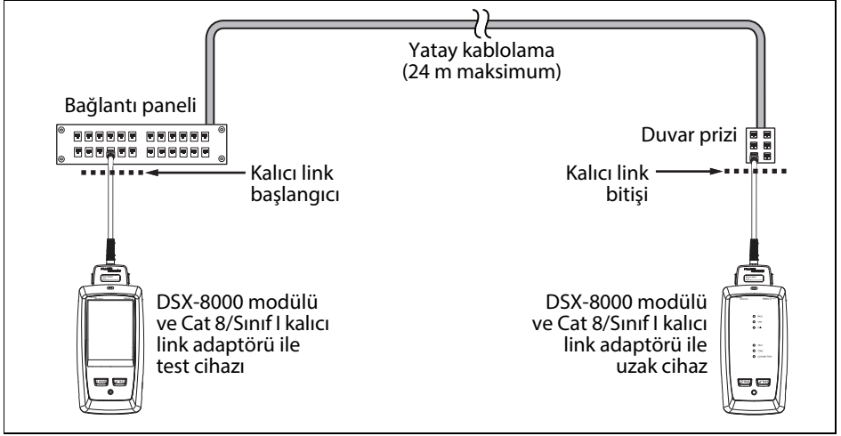
Şekil 3. Kalıcı Link Bağlantıları, Cat 8/Sınıf I Linkler için
