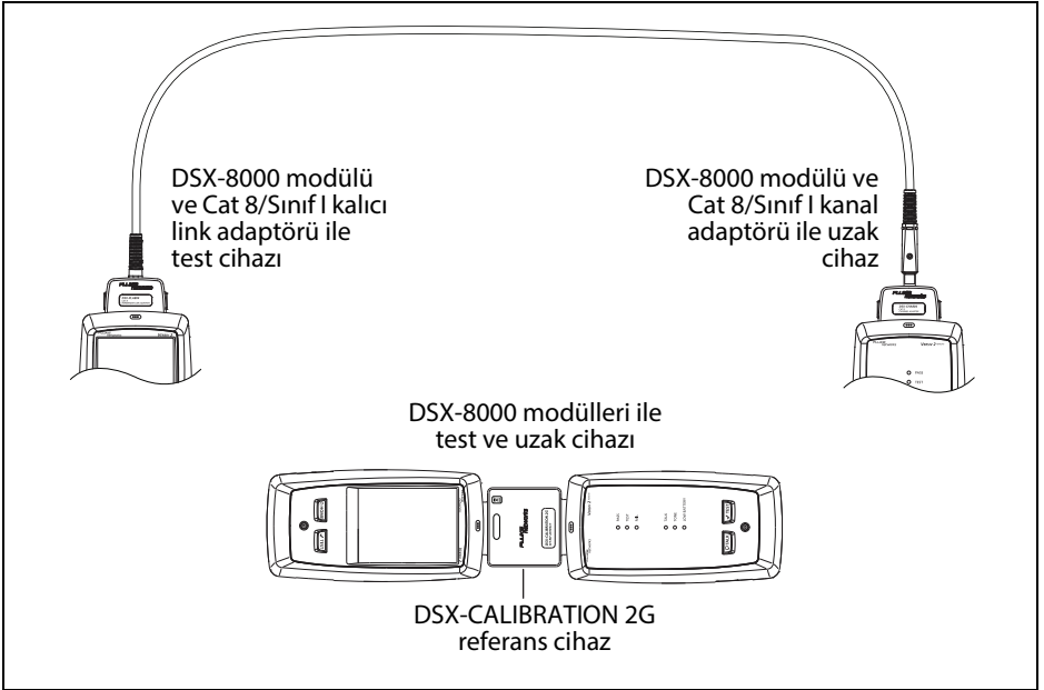
Şekil 2. Cat 8/Sınıf I Referans Bağlantıları
