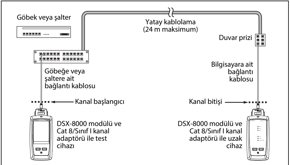
Şekil 4. Kanal Bağlantıları, Cat 8/Sınıf I Linkler için
