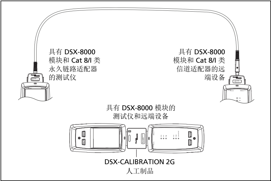
图 2. Cat 8/I 类测试限制的参照连接
