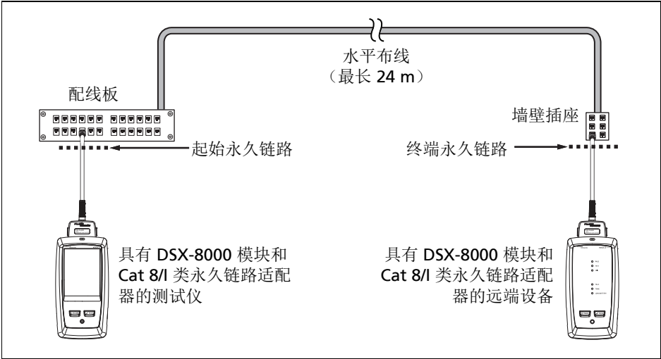
图 3. 用于 Cat 8/1 类链路的永久链路连接
