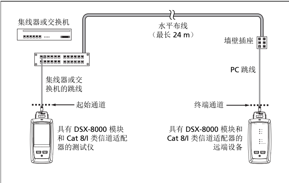
图 4. 用于 Cat 8/1 类链路的信道连接
