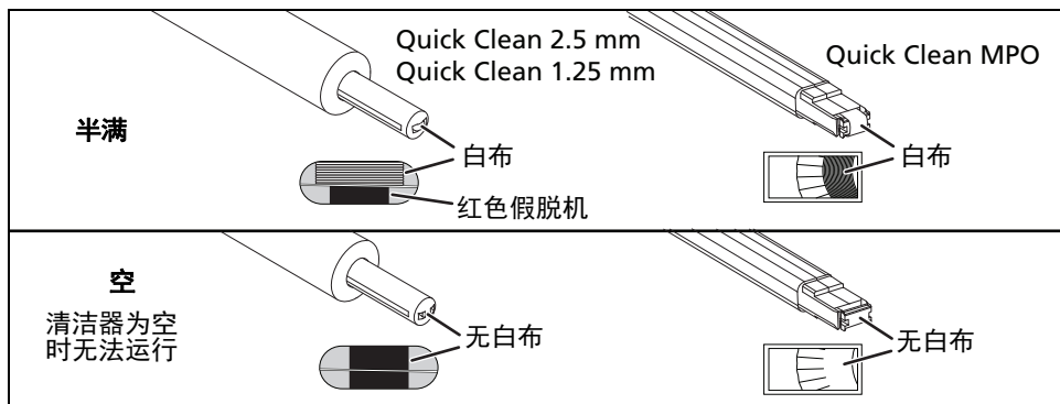
图 1. 显示清洁剂中有多少布的窗口
