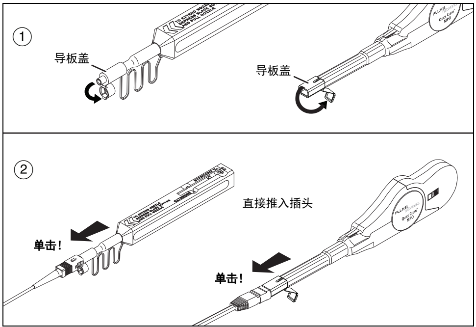
图 3. 如何清洁插头的端面
