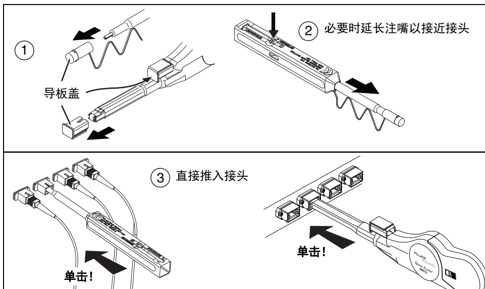
图 2. 如何清洁适配器的端面
