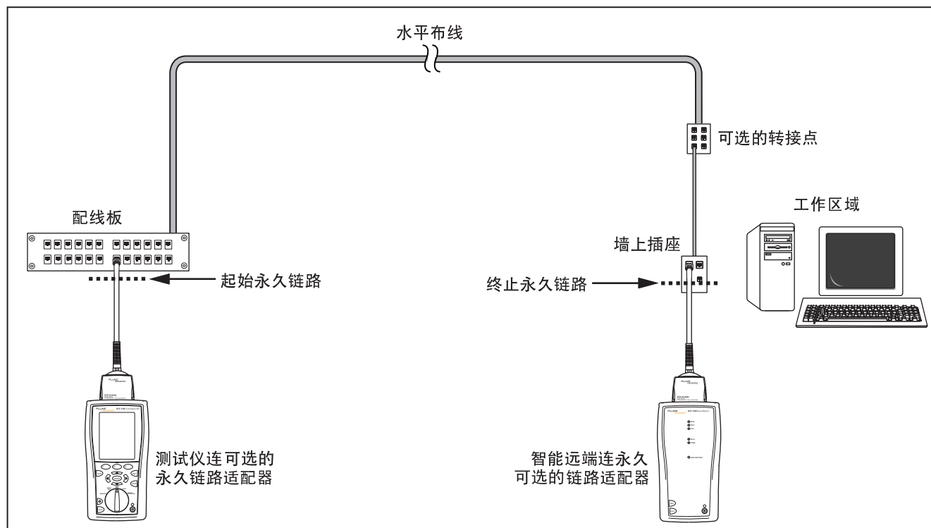
图 12. 永久链路测试连接
