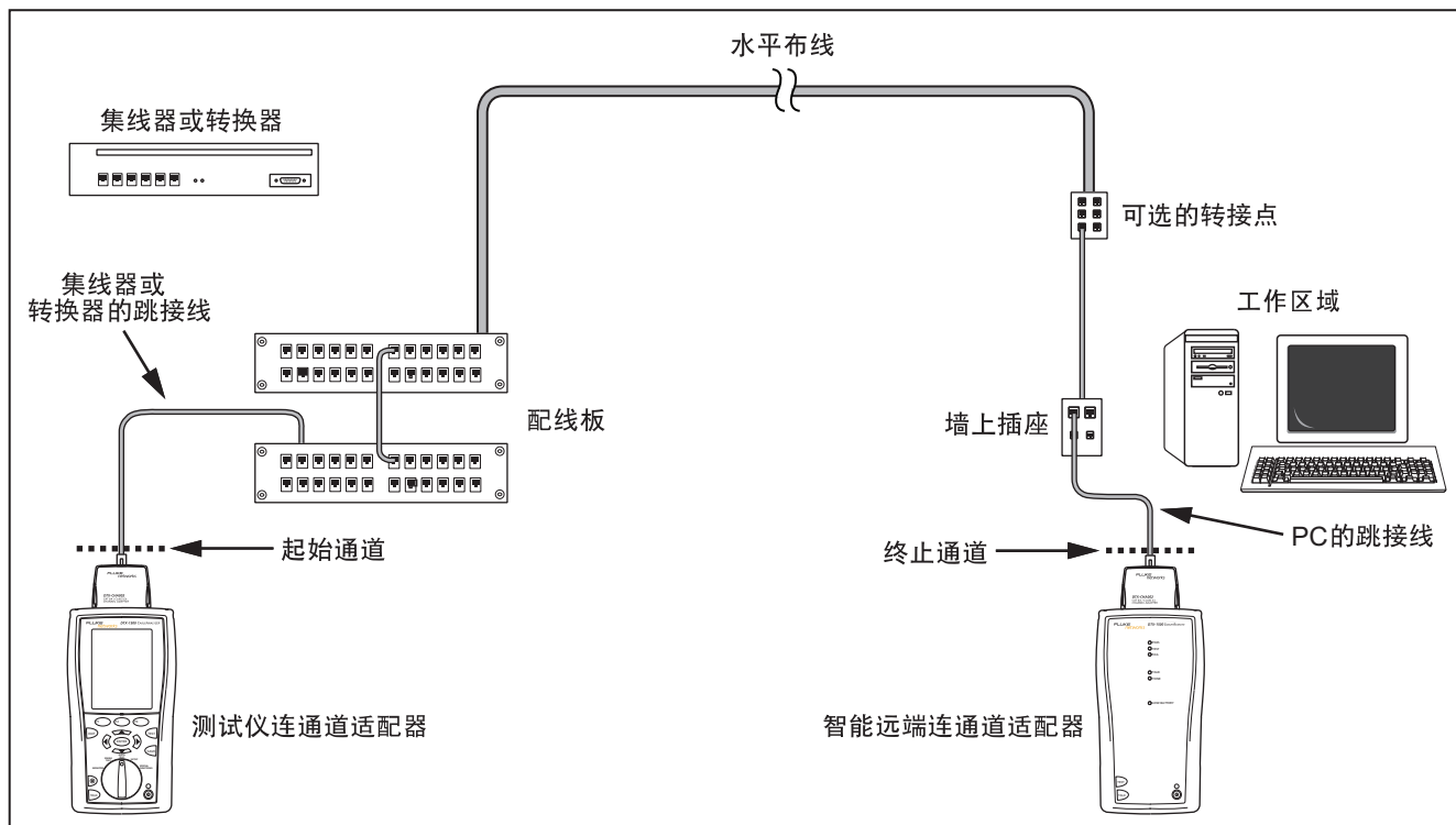
图 13. 通道测试连接
