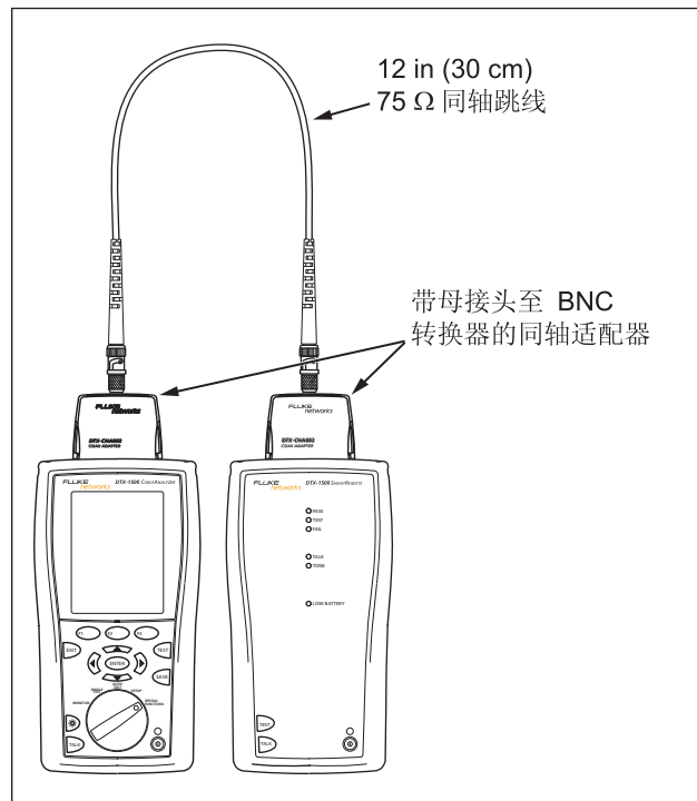
图 17. 同轴电缆基准连接
