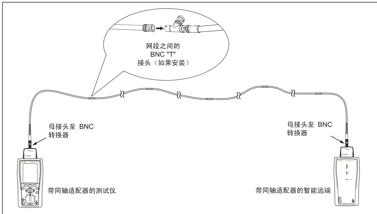
图 19. 同轴电缆网络布线测试连接
