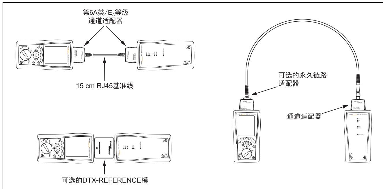
图 9. 双绞线基准连接
