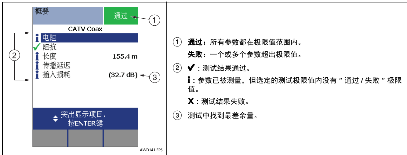
图 21. 同轴电缆布线自动测试结果
