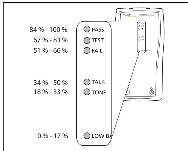
图 5. 启动后显示的智能远端电池状态
