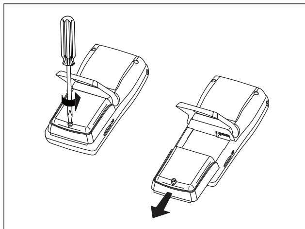
图 4. 拆卸电池组
