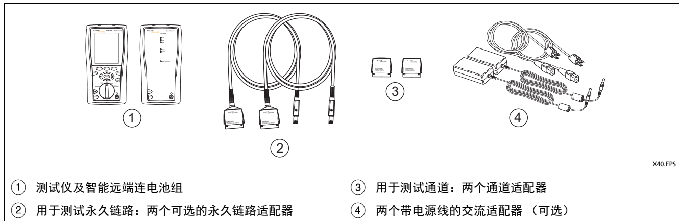
图 11. 认证双绞线布线所需的装置
