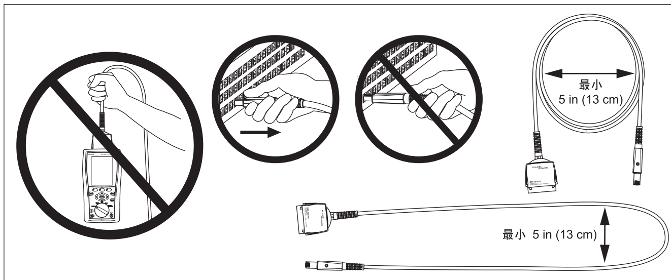
图 7. 可选的永久链路适配器使用指南
