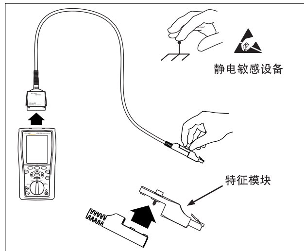
图 8. 更换可选的 DTX-PLA001 适配器上的特征模块
