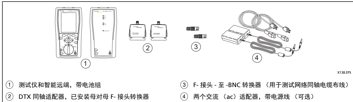
图 18. 同轴电缆布线认证设备
