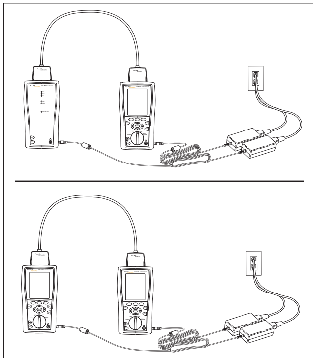
图 23. 用更新的测试仪更新软件
