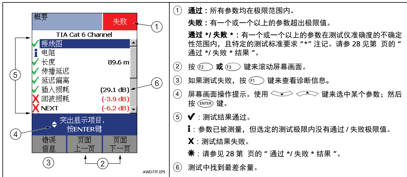
图 14. 双绞线布线自动测试概要
