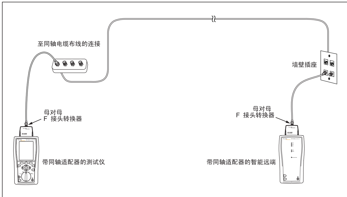
图 20. 同轴电缆视频布线测试连接
