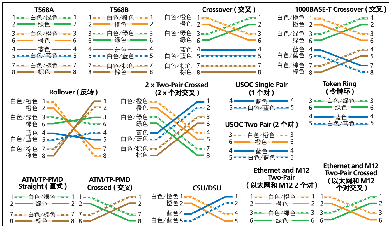
图 10. 插座配置
