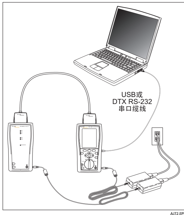
图 22. 用 PC 更新软件
