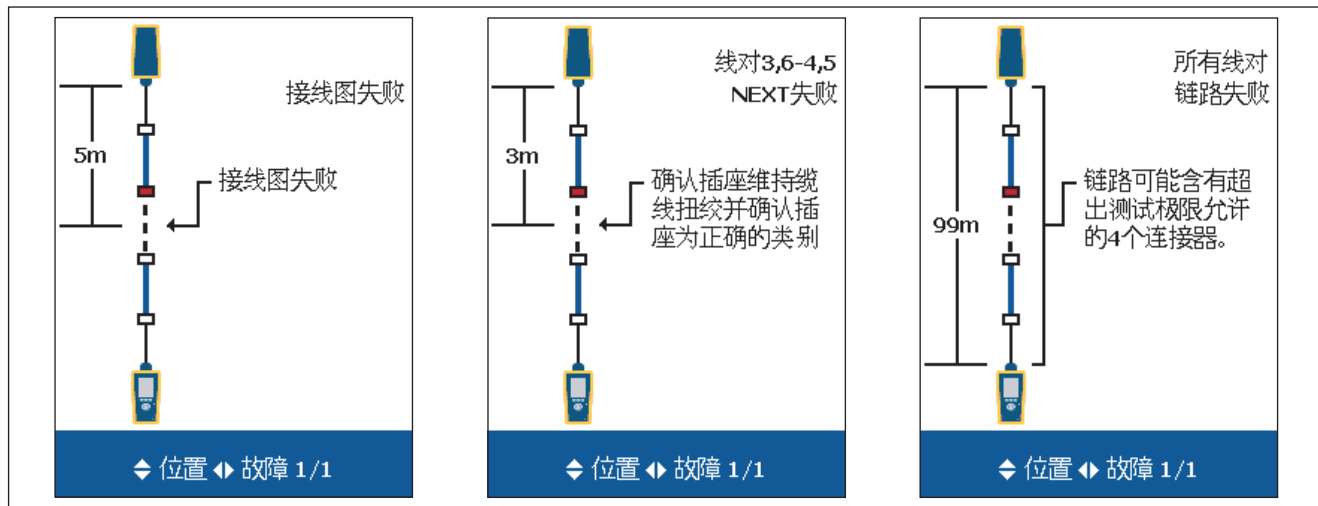
图 16. 自动诊断屏幕画面实例
