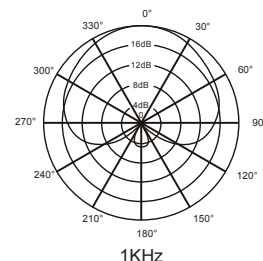
Richtcharakteristik
