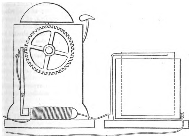
Fig. 19.—Cooke's Alarum.
