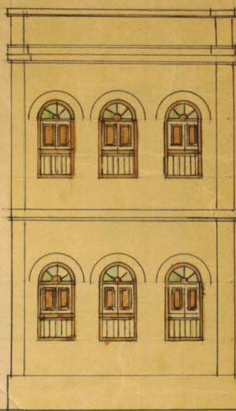
ELEVATION
