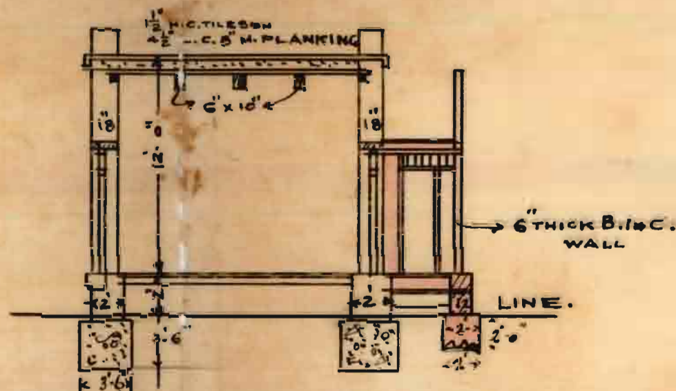
— CROSS SECTION A.B. —
