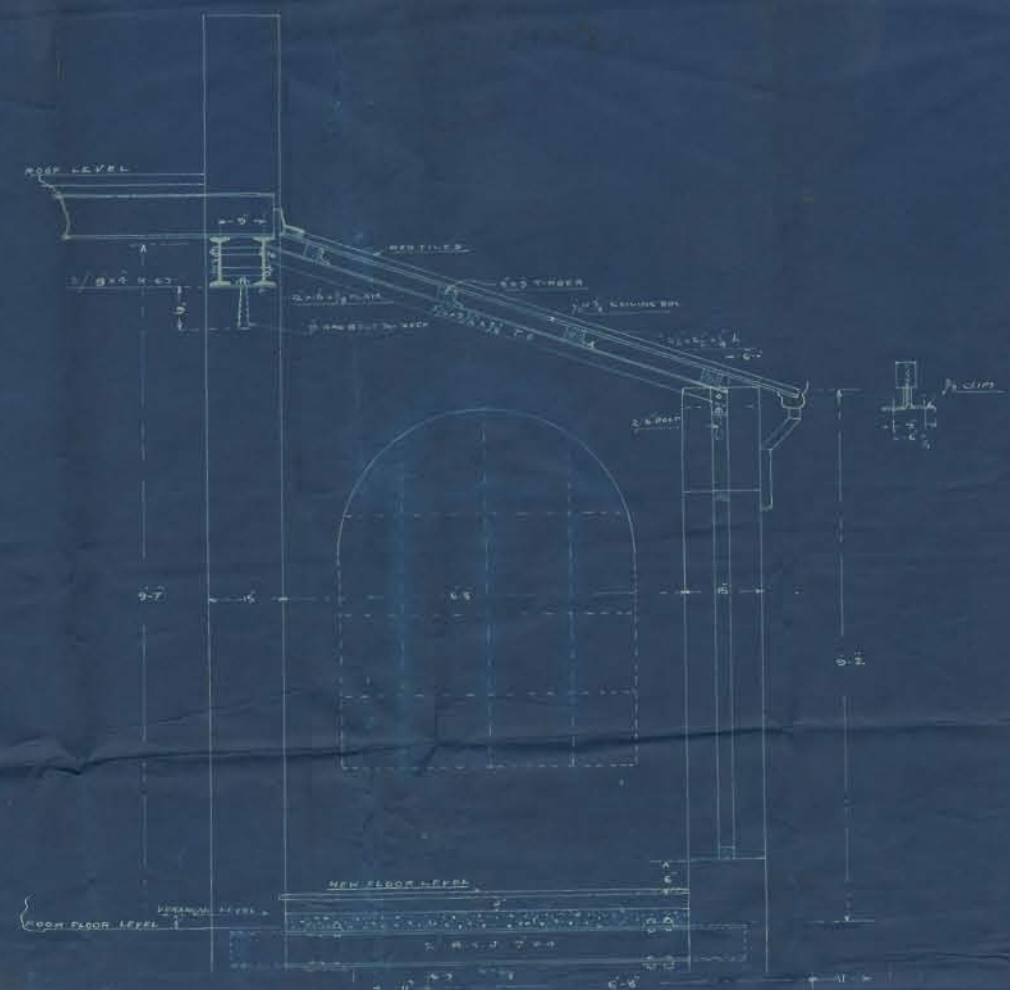
— SECTION CD — — NEW VERANDAH —
