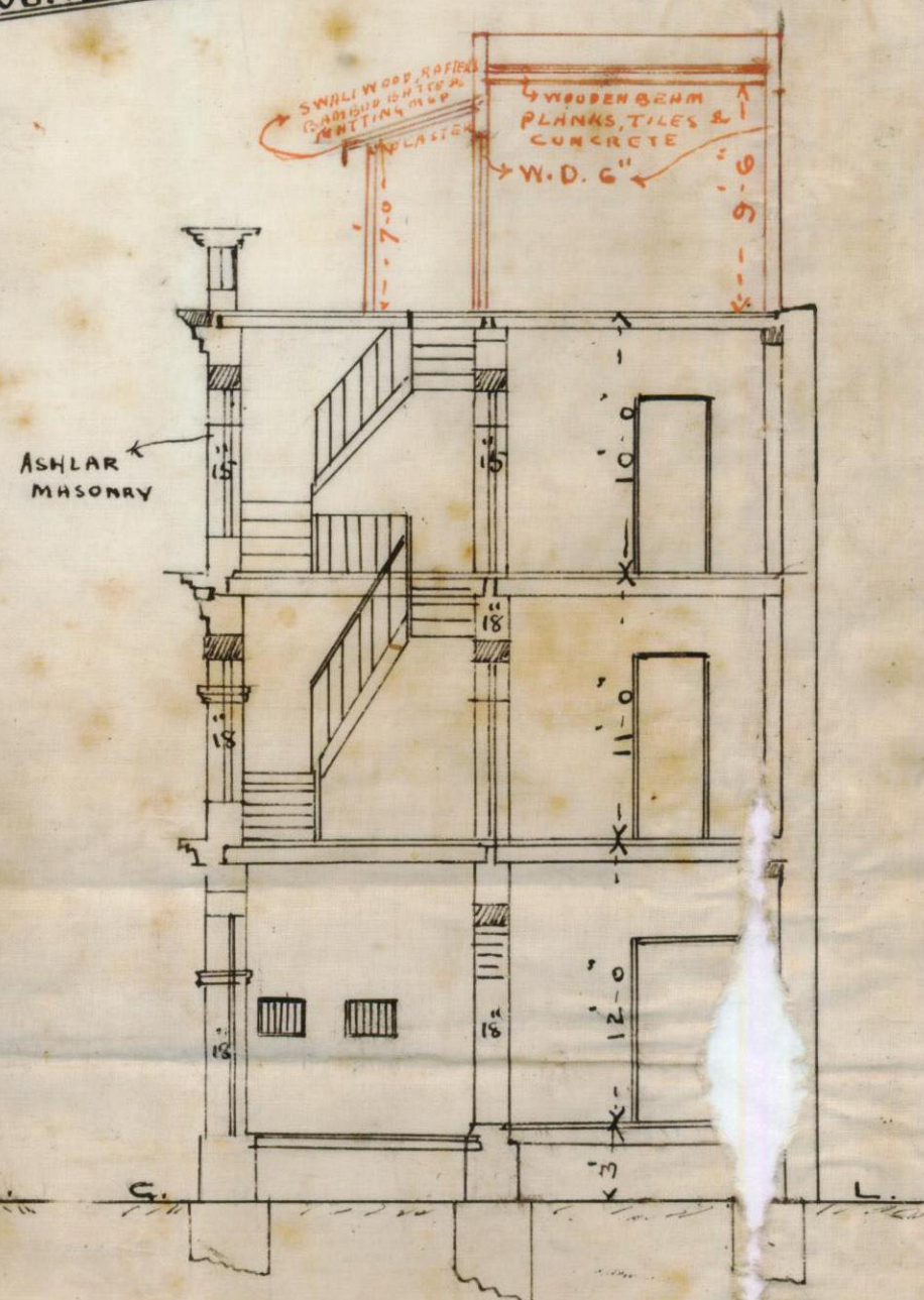
SECTION A-B
