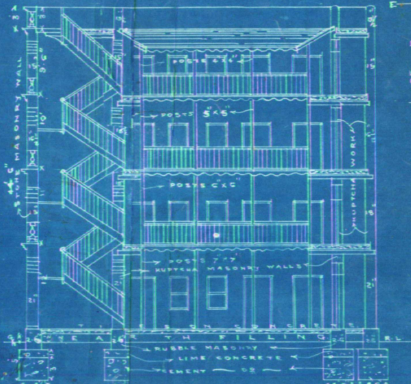
SECTION A-B.
