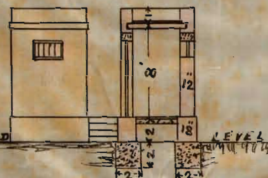
LONGITUDINAL SECTION ON GH
