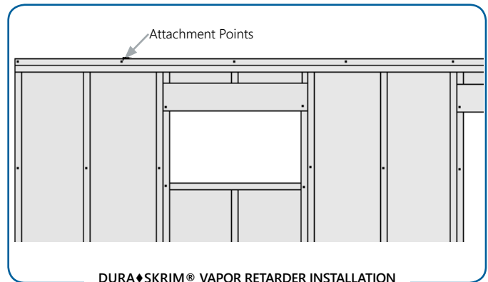
DURA♦SKRIM® VAPOR RETARDER INSTALLATION Metal Studs
