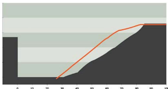
Profil du versoir N° 28 comparé au N° 9 Profondeur de travail : 26 cm, en bas : 30 cm, largeur 73 cm
