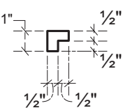
Sliding Door Frame (x2) Scale 1:100
