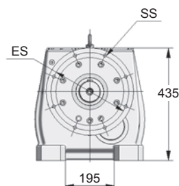
Vista lado da saída
