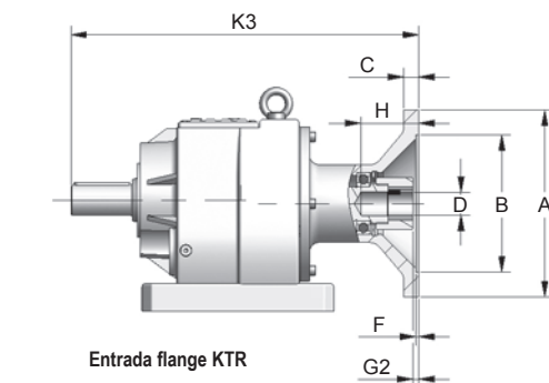
Flange Lanterna / KTR
