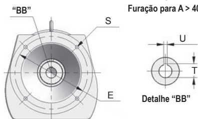
Furação para A > 400
