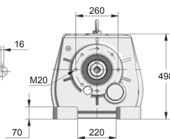
Vista lado da saída
