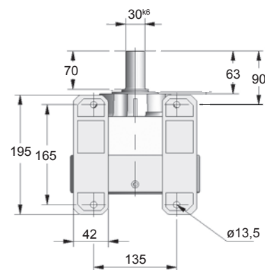
Detalhe dos pés
