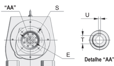
Vista lado da entrada
