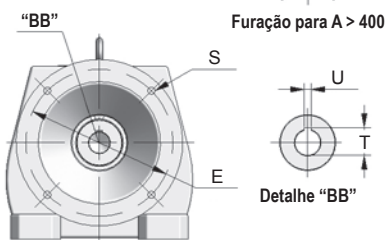
Furação para A > 400
