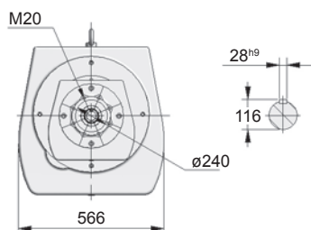
Vista lado da entrada
