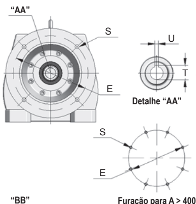
Furação para A > 400
