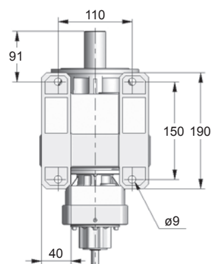
Detalhe dos pés
