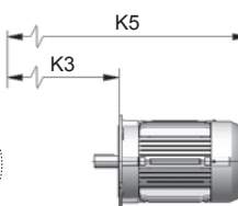
Entrada flange KTR + motor standard*
