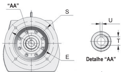
Vista lado da entrada
