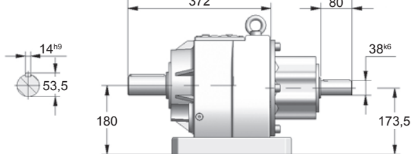
Entrada eixo integral
