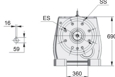
Vista lado da saída
