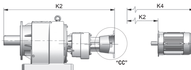
Entrada flange lanterna
