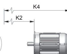
Entrada flange lanterna
