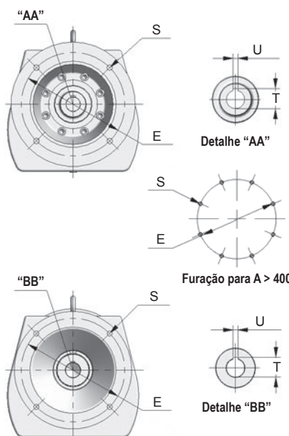
Vista lado da entrada
