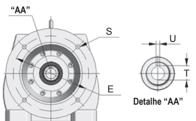
Vista lado da entrada
