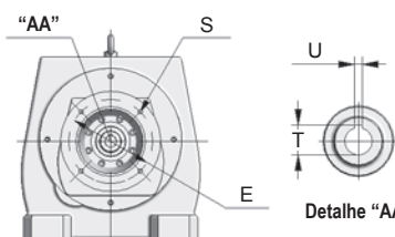
Vista lado da entrada
