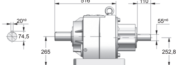
Entrada eixo integral
