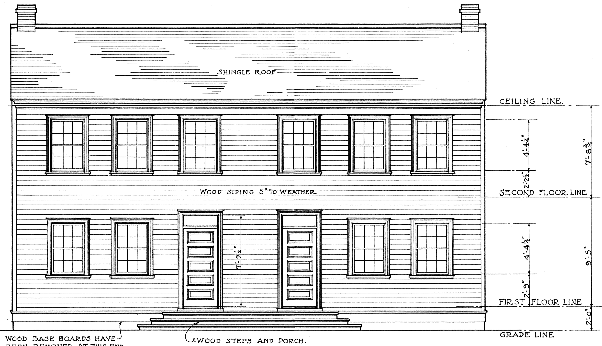
· EAST · ELEVATION ·
