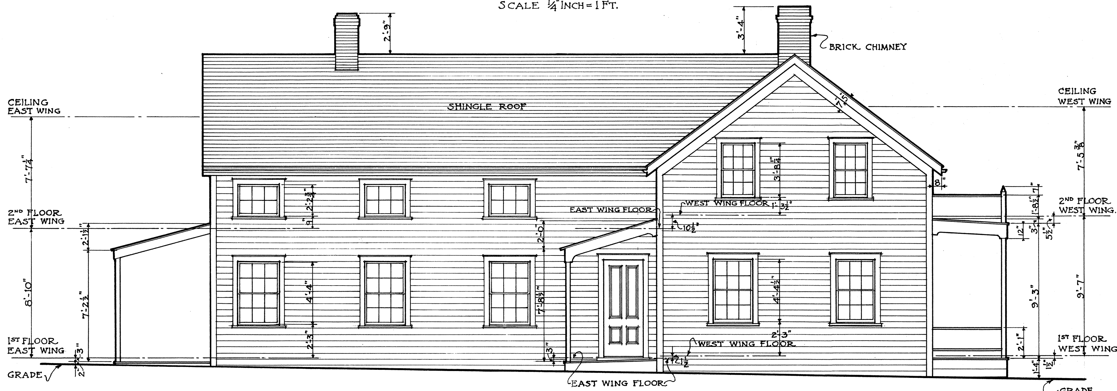
· NORTH · ELEVATION ·
