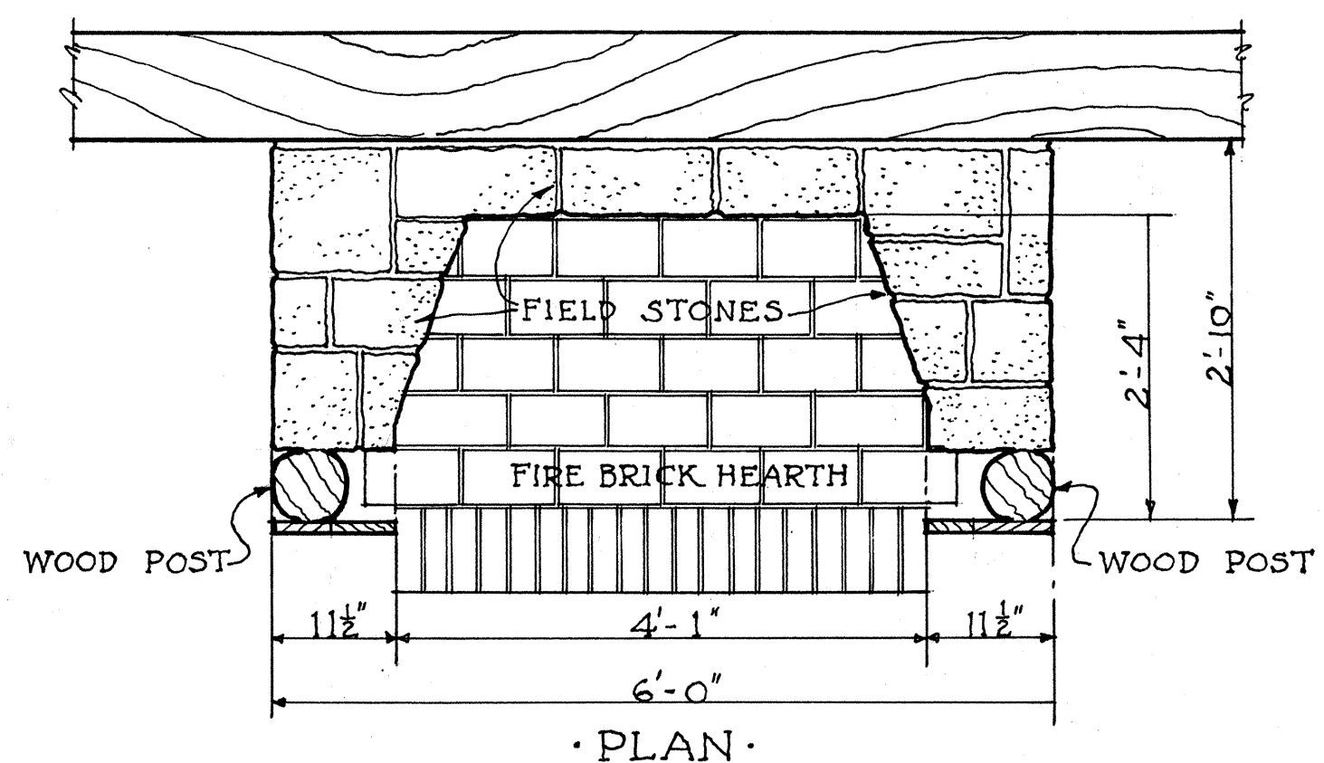
· 3/4" SCALE FIREPLACE DETAILS ·
