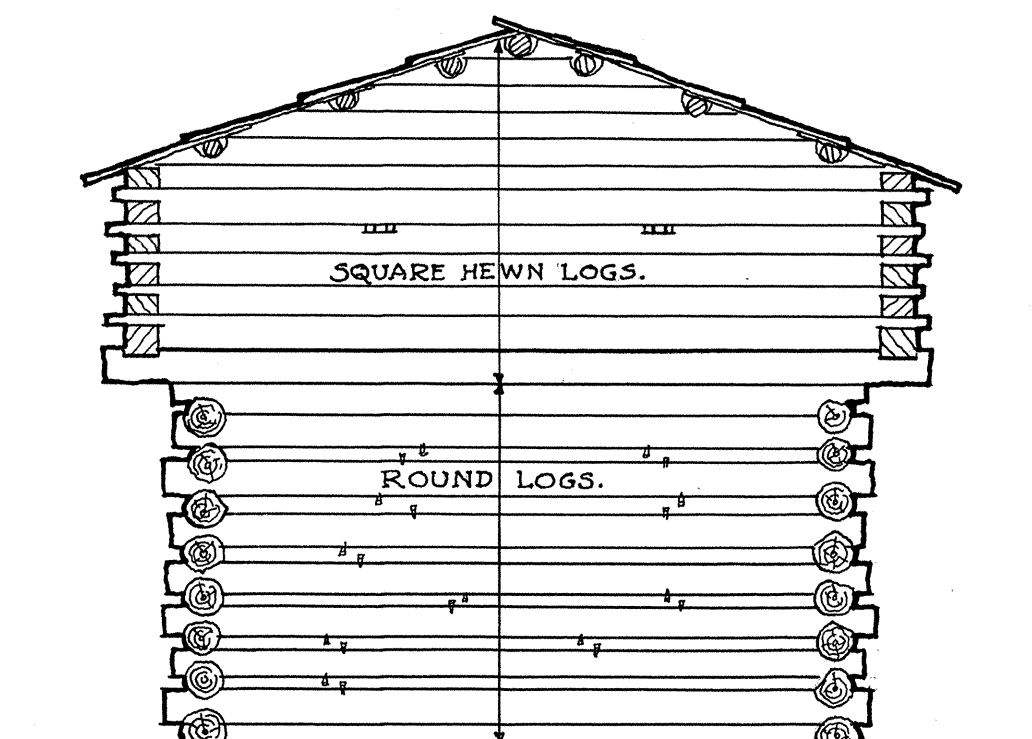
· NORTHEAST · ELEVATION ·
