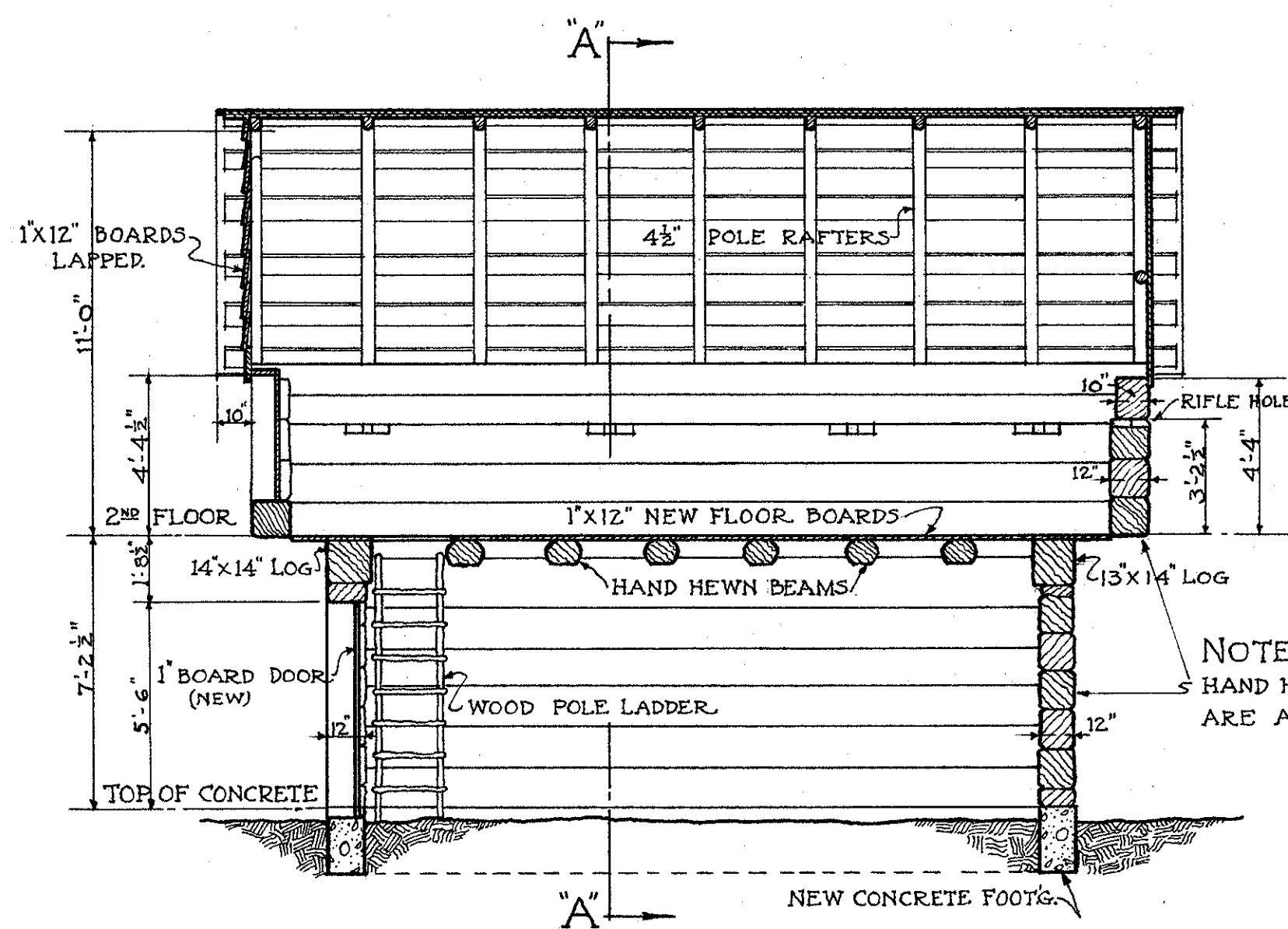
· LONGITUDINAL · SECTION · AT · "A-A" · SCALE \frac{1}{4}" = 1 \text{ FT.}
