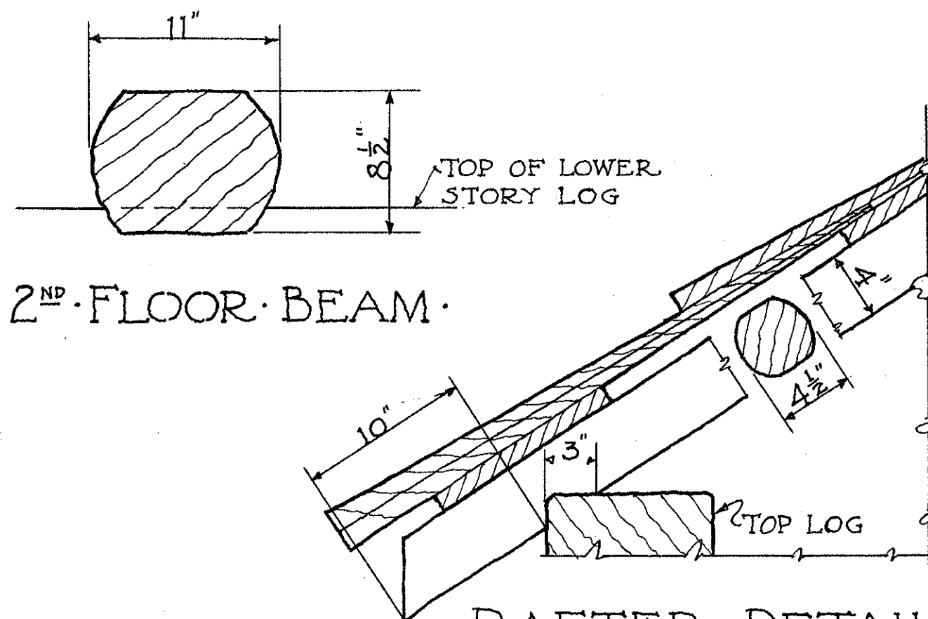
· RAFTER · DETAIL · SCALE 1\frac{1}{2}" = 1'-0"
