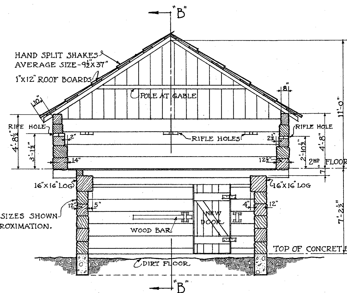
· CROSS · SECTION · AT · "B-B" · SCALE \frac{1}{4}" = 1 \text{ FT.}
