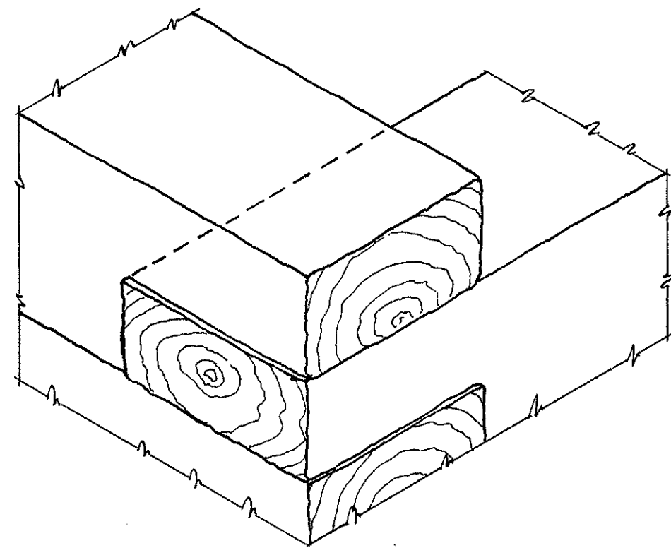
· DETAIL · OF · LOG · JOINT · SCALE 1\frac{1}{2}" = 1'-0"
