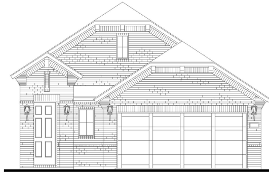
Elevation B
