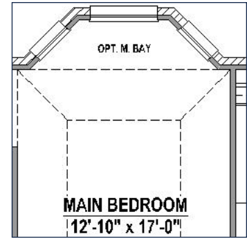
Optional Main Bay (+27 SF)
