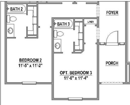
Optional Bedroom 3 & Bath 3 (+105 SF)
