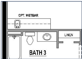
Optional Wet Bar
