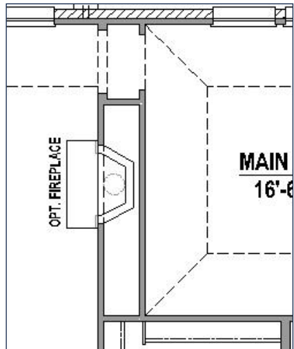
Optional Fireplace
