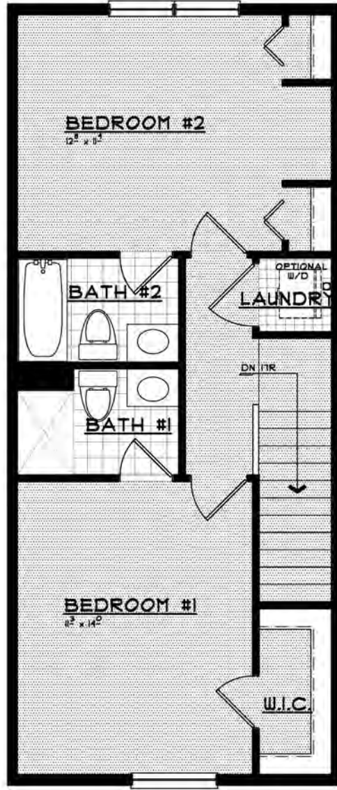
Optional Layout
