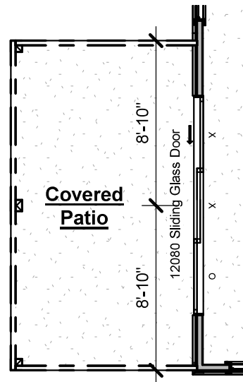
12' Sliding Door
