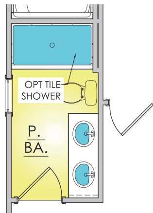
4 - OPTIONAL TILE SHOWER
