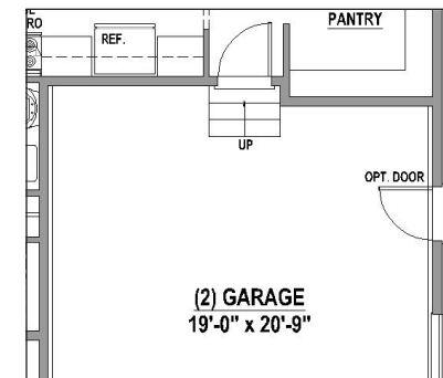
Optional Garage Service Door
