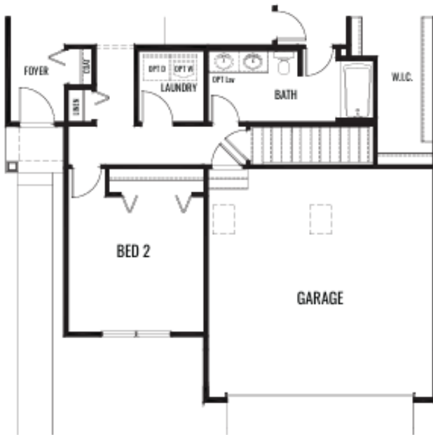
OPTIONAL BASEMENT
