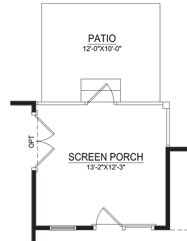
OPTIONAL SCREEN PORCH
