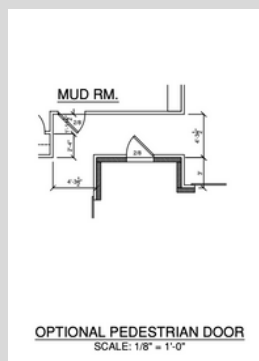
OPTIONAL PEDESTRIAN DOOR
