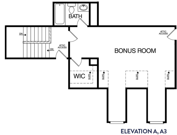
ELEVATION A, A3
