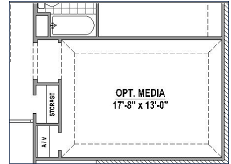
Optional Media Room (+270 SF)
