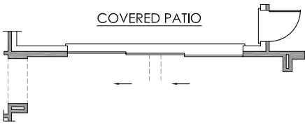
15080 3-PANEL MULTI-SLIDING DOOR OPT.
