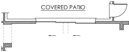
12080 3-PANEL MULTI-SLIDING DOOR OPT.
