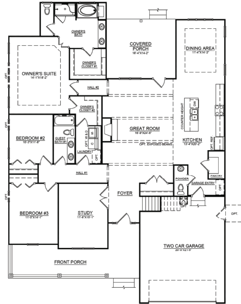
OPTIONAL GUEST BATH #1
