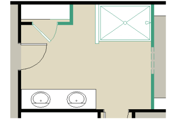
OPTIONAL TILE SHOWER
