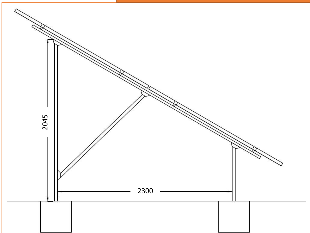
Vista Lateral
