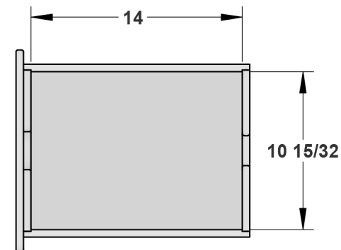
TYP. DRAWER
