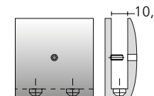
opa 600 w 49 x h 49 x d 22mm w 1,93 x h 1,93 x d 0,87"
