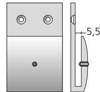
opa 100 w 49 x h 79 x d 17mm w 1,93 x h 3,11 x d 0,67"
