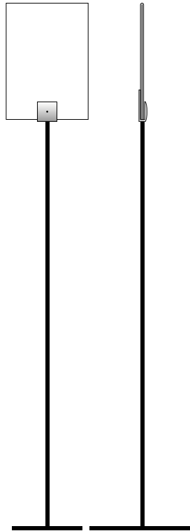
opa 900 A4 w 210 x h 1347 x d 270mm (A4 : w 210 x h 297mm) w 8,27 x h 53,03 x d 10,63" (w 8,27 x h 11,69")
