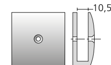
opa 700 w 49 x h 49 x d 22mm w 1,93 x h 1,93 x d 0,87"
